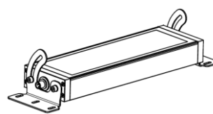
HERIONOVA.FX01 Montážní držáky z nerezové oceli tloušťky 2 mm – 45° rotace.
